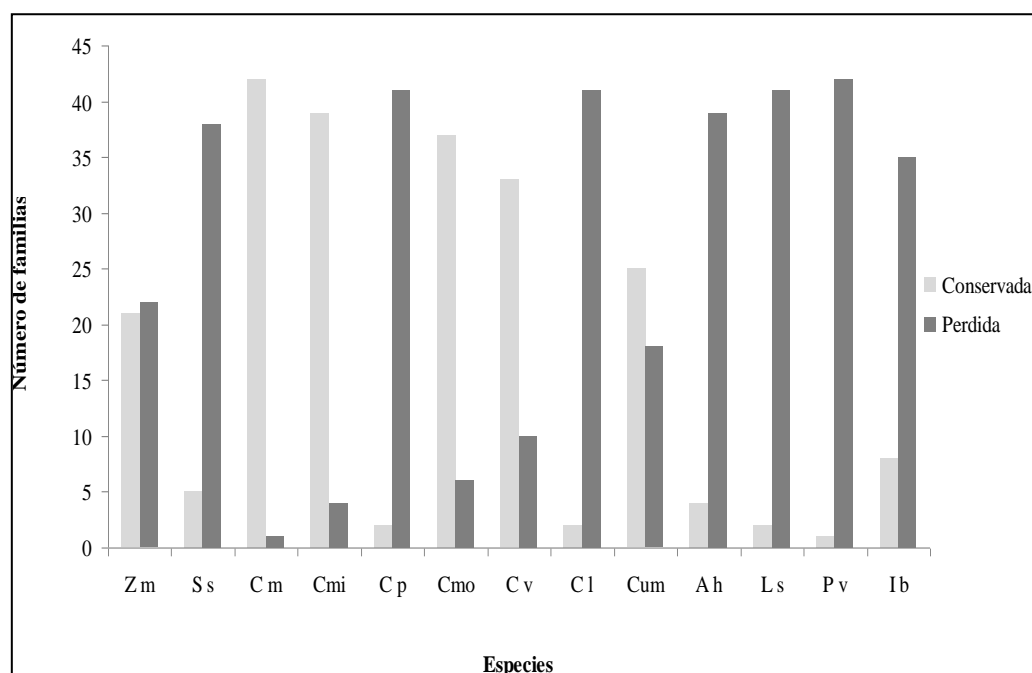
FIGURA 2. Frecuencia de conservación de especies por familias en el territorio. Zm ( Z. mays ), Ss ( S. sacharum ), Cm ( C. maxima ), Cmi ( C. mixta ), Cp ( C. pepo ), Cmo ( C. moschata ), Cv ( C. vulgaris ), Cl ( C. lanatus ), Cum ( C. melo ), Ah ( A. hypogea ), Ls ( Lagenaria siceraria ), Pv ( Phaseolus vulgaris ), Ib ( Ipomea batatas ). Cm (zapallo), Cmi (calabaza), Cmo (anco), Cv (sandía): resultan las más conservadas por las familias.-Ss (caña dulce): perdieron la mayoría de las familias. Al igual que Cp=Cl=Ah=Ls=Pv=Ib.
