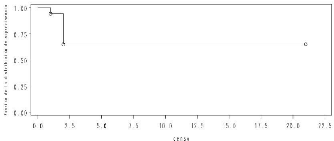
FIGURA 2. Representación gráfica de la supervivencia de plántulas de B. bipinnata evaluada en tres épocas del año en sierra de Huautla Morelos, México. 2015.
