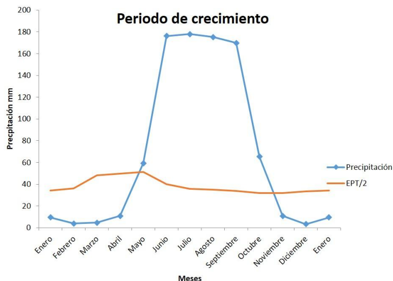
FIGURA 1. Periodo de crecimiento en “Camino a Pizotlan” en base a la estación meteorológica de Tepalcingo Morelos. México 2015.
