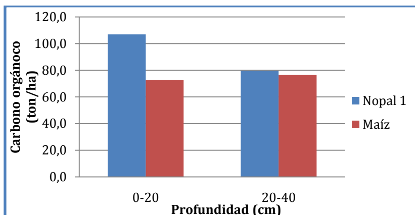
FIGURA 2. Valor (ton/ha) de los niveles de carbono orgánico de suelos promedio para el cultivo de nopal y maíz a profundidades de 0-20 y 20-40 cm.
